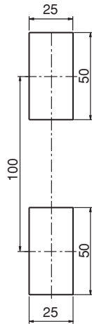
Монтажное отверстие
