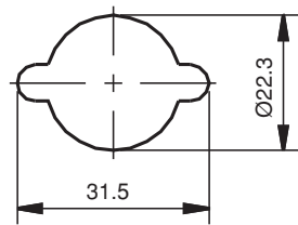
Монтажное отверстие
