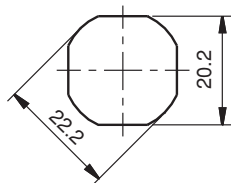
Монтажное отверстие
